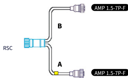
D10513 A: 3,5 m / B: 3,5 m 16V
